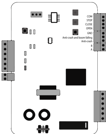
Conexión de la terminal U1000/U2000 con la barrera vehicular.
